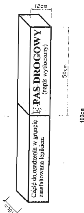
Rysunek 1. „Świadek” do wyznaczenie pasa drogowego
