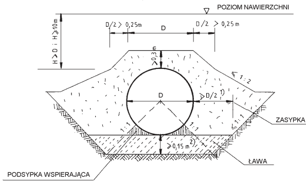
Rys. 8. Zasyпка nad przepustem jednorurowym
