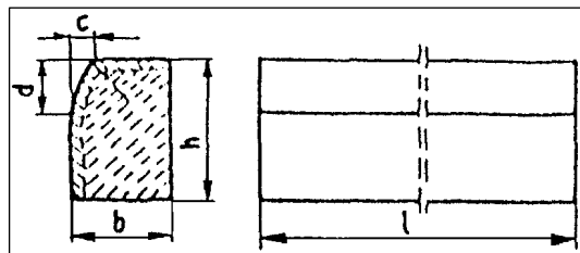
Rys. 1. Wymiarowanie krawężników i oporników
