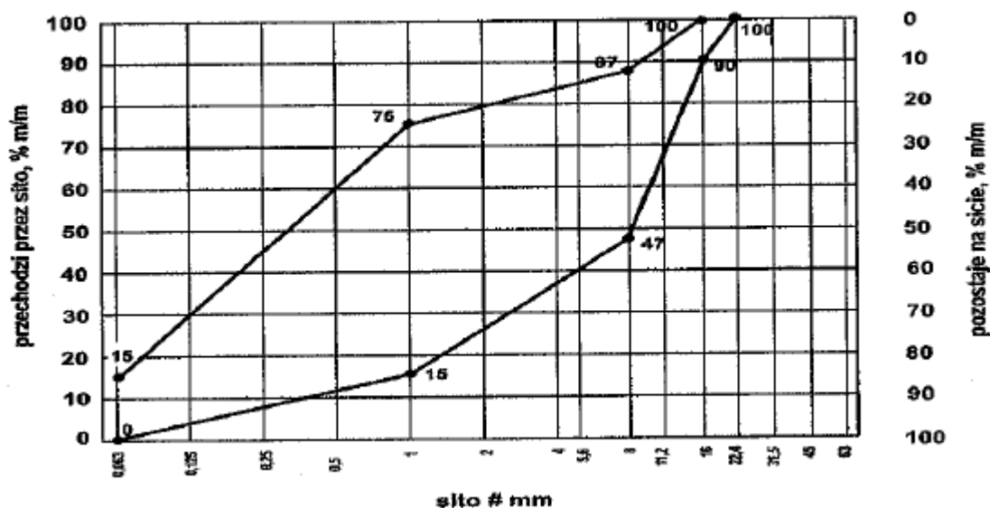
Rysunek 1. Mieszanka niezwiązana 0/16 do warstwy ulepszanego podłoża stabilizowanego georusztem
